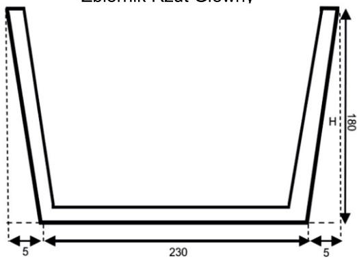
Zbiornik Rzut Główny
