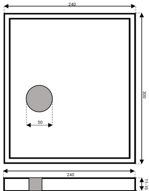
Pokrywa Zbiornika Rzut Poziomy
