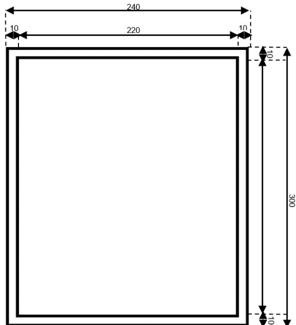
Zbiornik Rzut Poziomy
