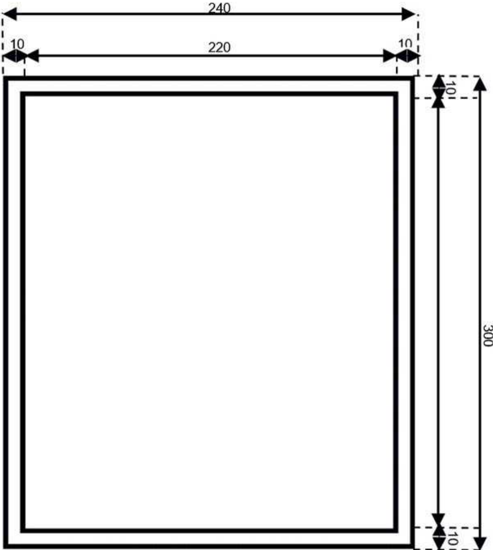
Zbiornik Rzut Poziomy
